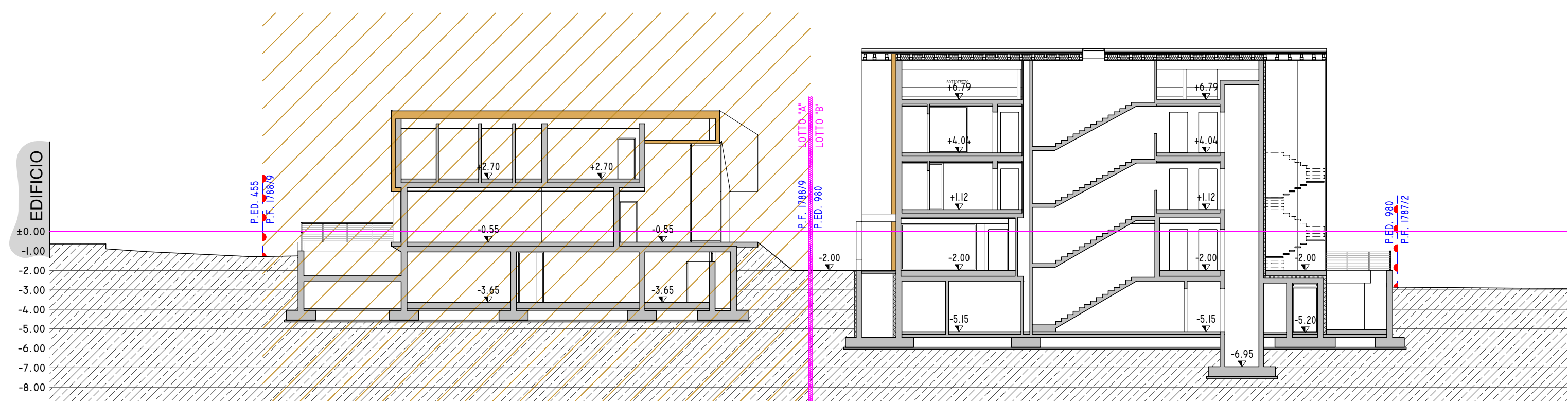
SEZIONE 3-3
