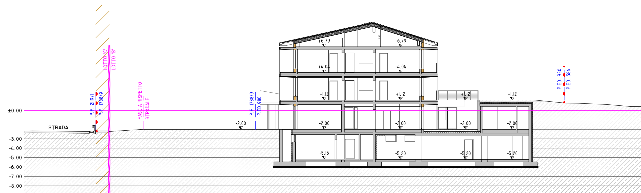
SEZIONE 2-2
