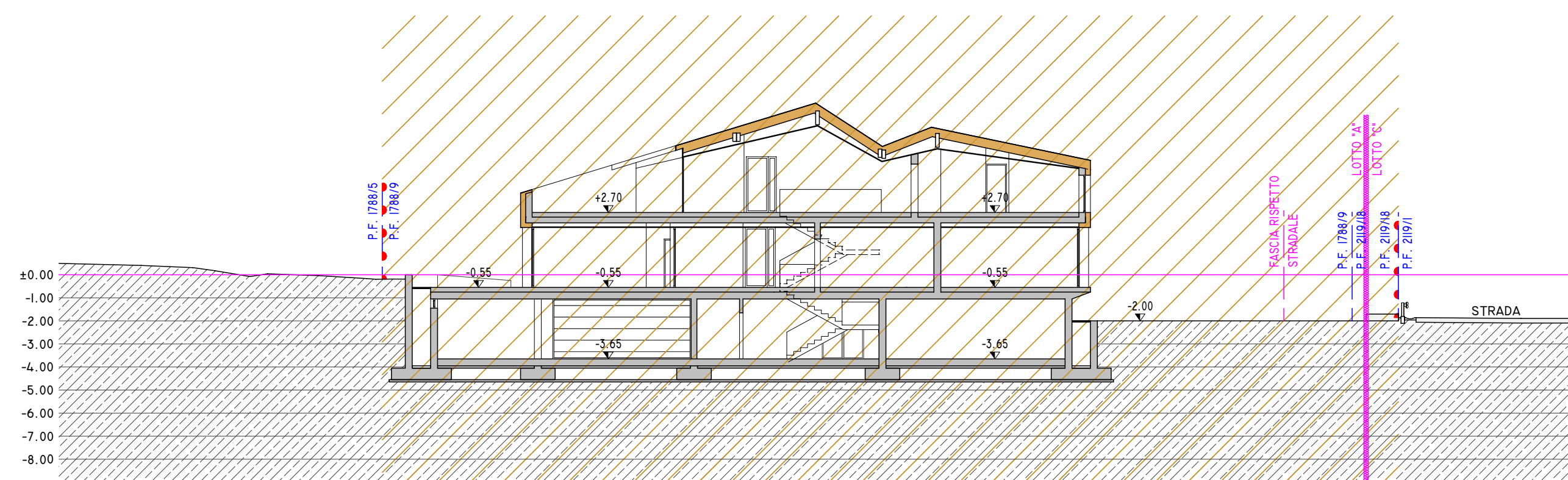
SEZIONE 1-1
