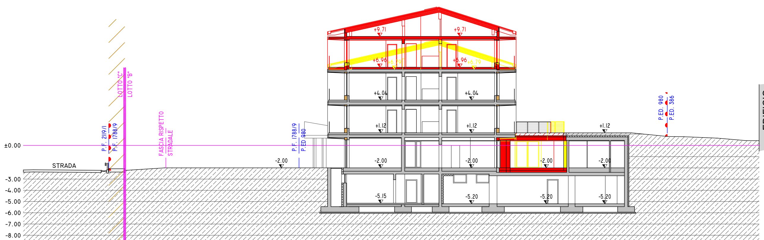
SEZIONE 2-2
