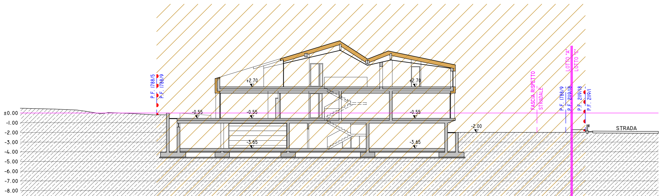
SEZIONE 1-1
