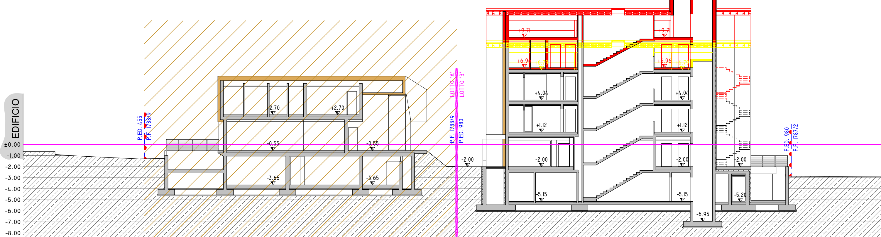
SEZIONE 3-3
